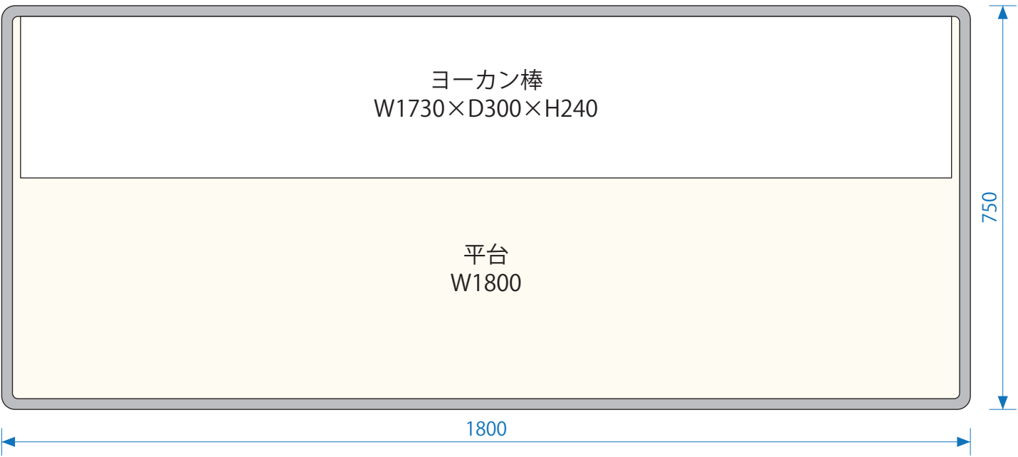
平面図
