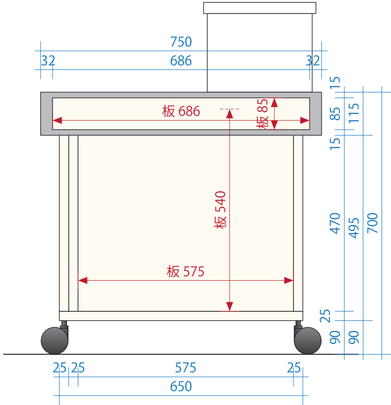
側面図
