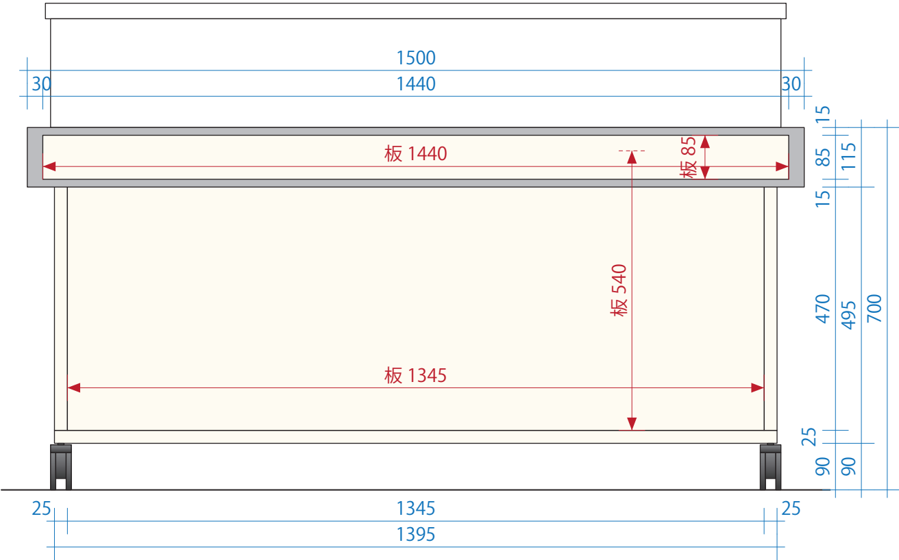
正面図
