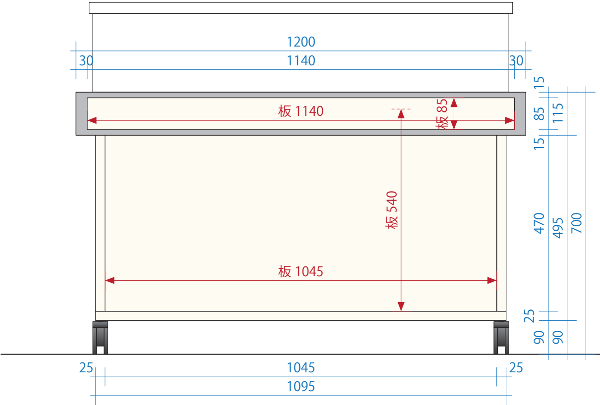
正面図
