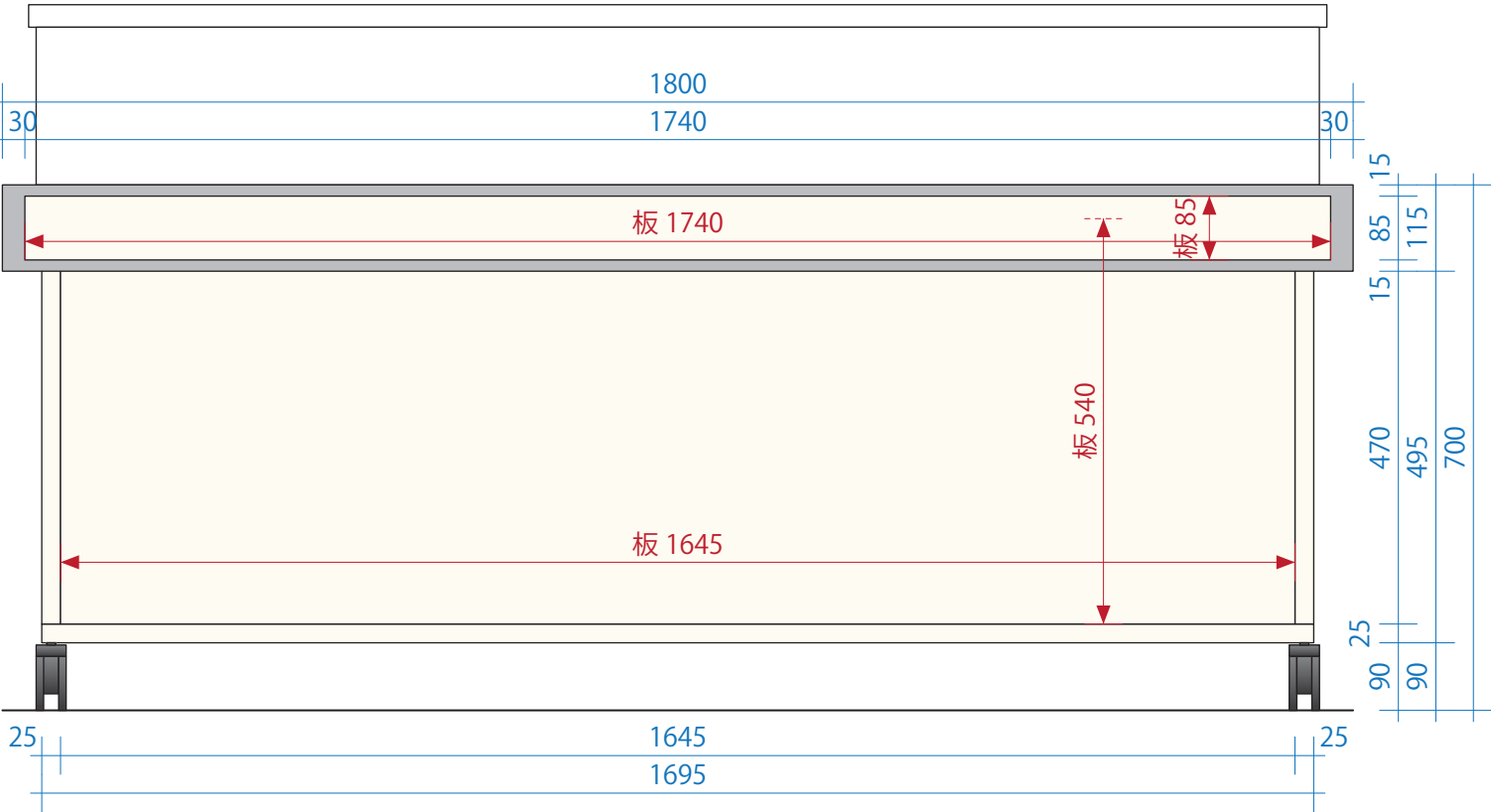
正面図
