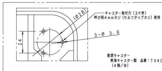
キャスター取付 参考寸法図
