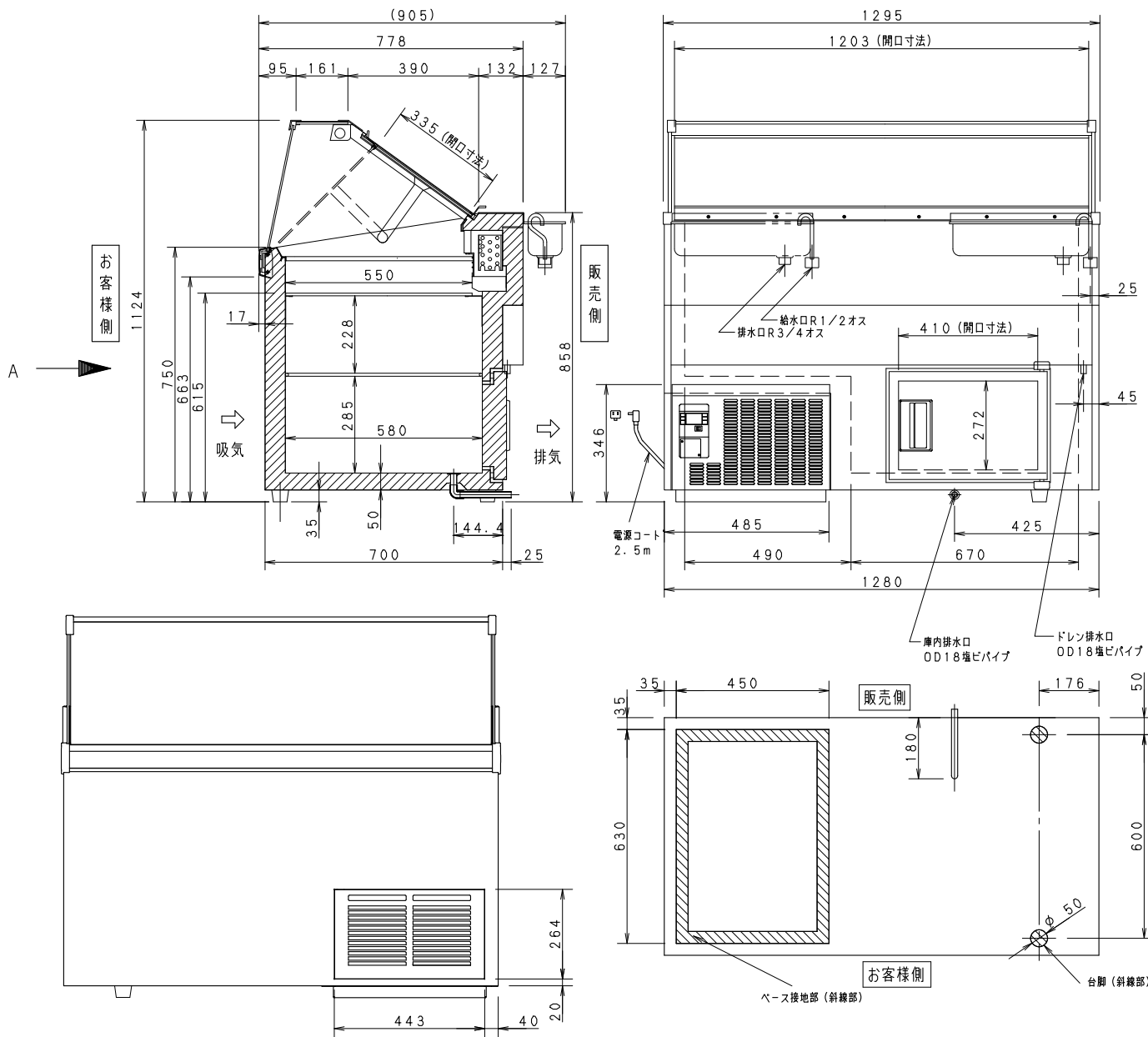
A矢視（吸気パネル寸法）
