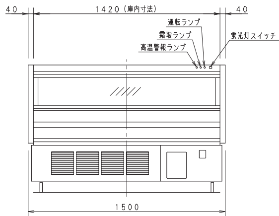
正面図
