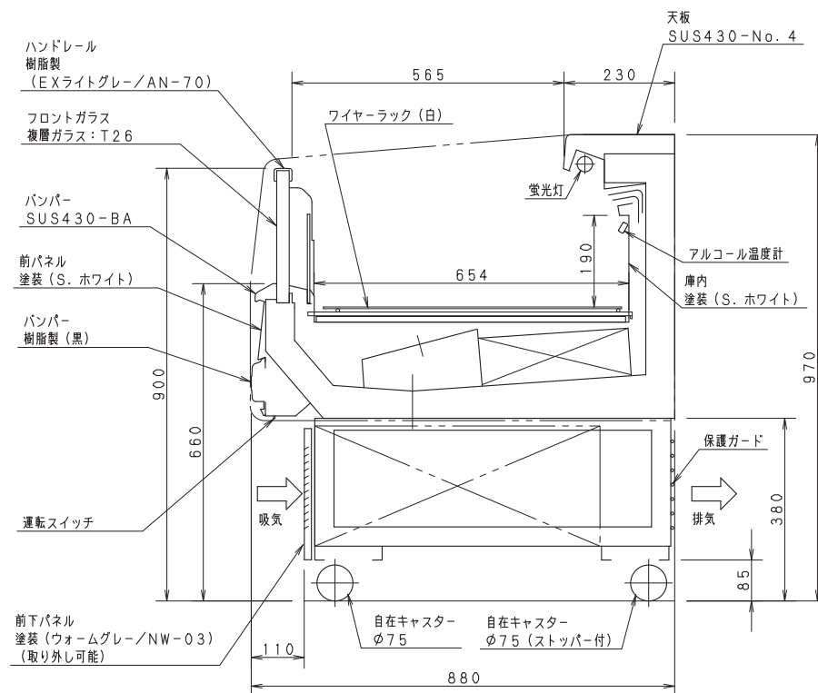
側面図
