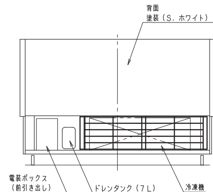
背面図
