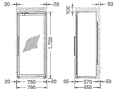
据付必要寸法図
